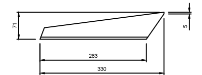
PIÈCE 18
