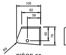
PIÈCE 20
