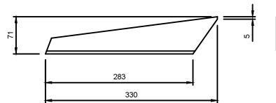
PIÈCE 17
