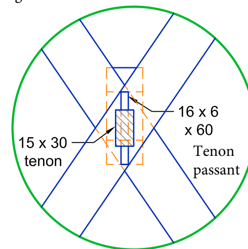
Détail 2 Échelle 1:3
