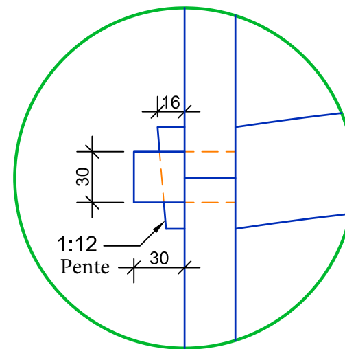
Détail 1 Échelle : 1:3
