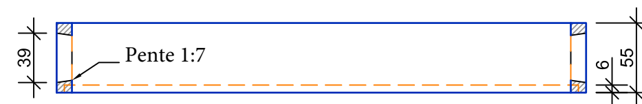
DÉTAIL DU TIROIR - NIVEAU SECONDAIRE
