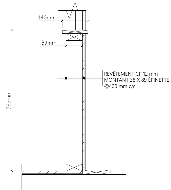
COUPE MUR NAIN ÉCHELLE 1:10
