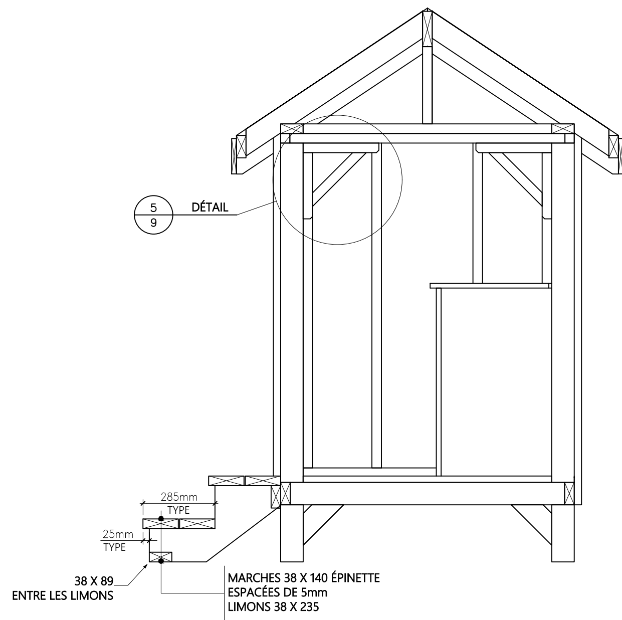
COUPE C-C ÉCHELLE 1:15
