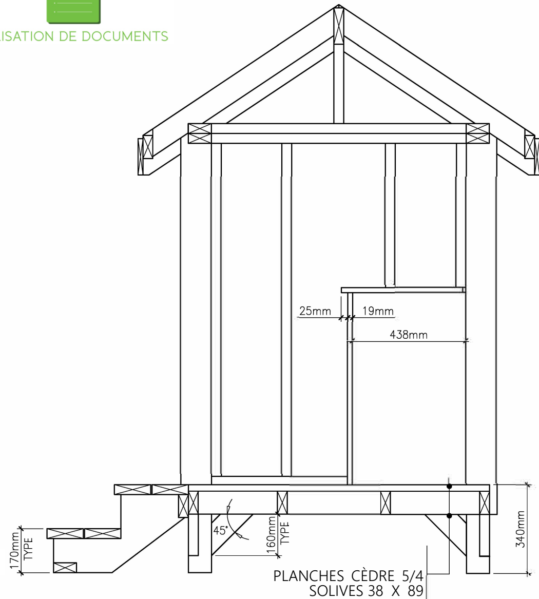
COUPE A-A ÉCHELLE 1:15
