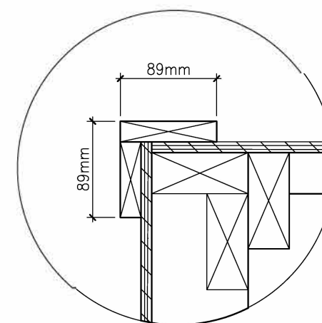
DÉTAIL 1 DÉTAIL BOISERIES DE COIN 2 TYPE
