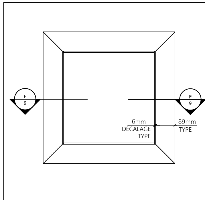
DÉTAIL DE LA FENÊTRE ÉCHELLE 1:10
