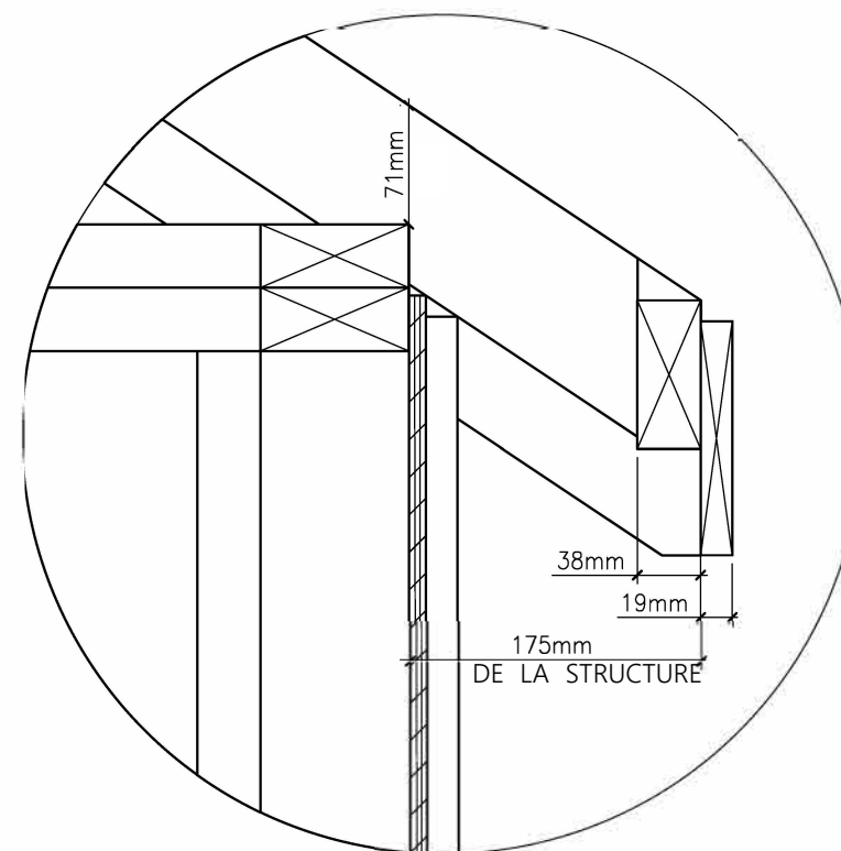
DÉTAIL 4 DÉTAIL DE L'AVANT-TOIT 6
