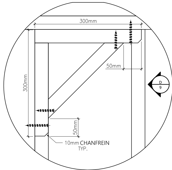
DÉTAIL ÉQUERRE ARCHITECTURALE ÉCHELLE 1:5
