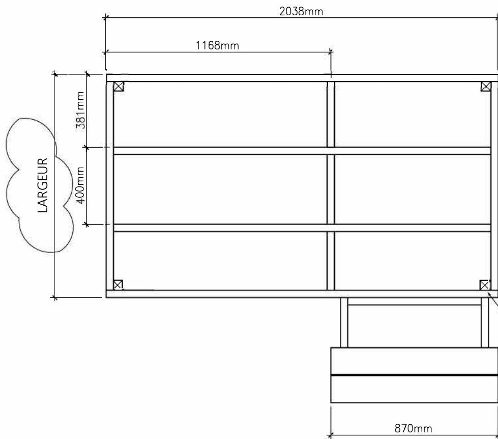
CHARPENTE DU PLANCHER
