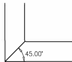
DÉTAIL DE LA SABLIÈRE INFÉRIEURE AU POTEAUX VU DU COIN GAUCHE DE L'ÉLEVATION AVANT ÉCHELLE 1:10
