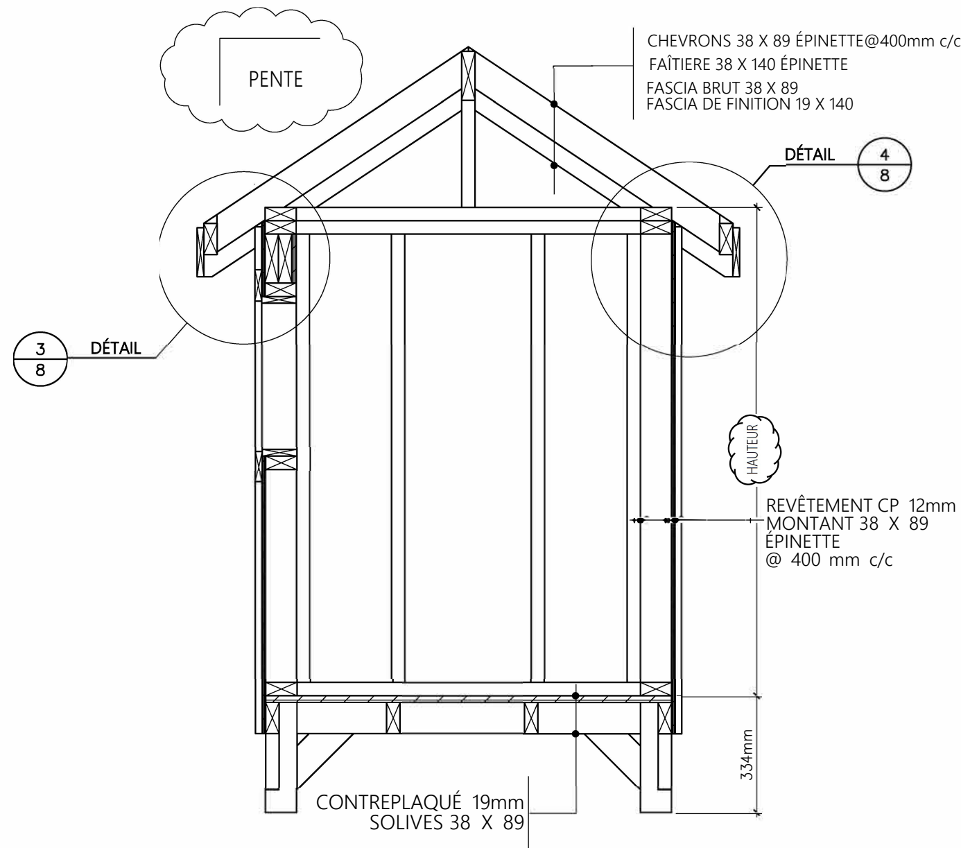
COUPE B-B ÉCHELLE 1:15
