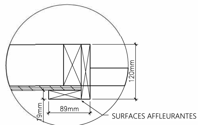
DÉTAIL 2 DÉTAIL BOISERIE 2 EXTRÉMITÉS MURS TYPE
