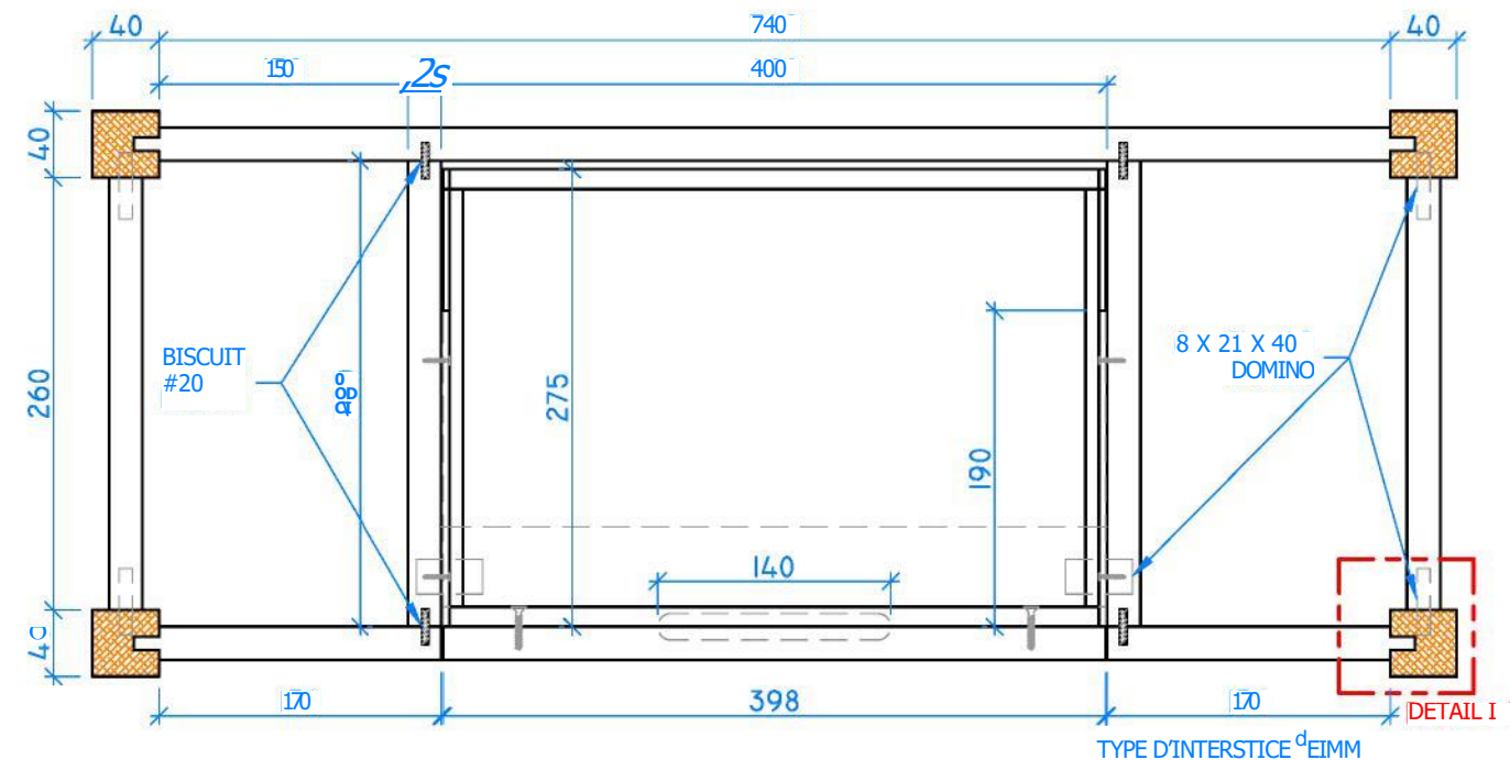
SECTION A : A ÉCHELLE 1 : 5
