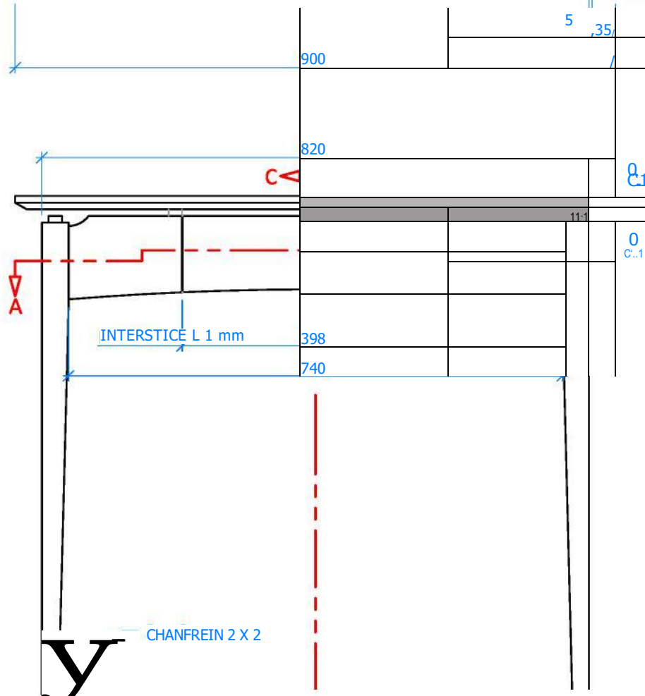
VUES DU DESSUS, DU DEVANT ET DU CÔTÉ DROIT ÉCHELLE 1 : 8
