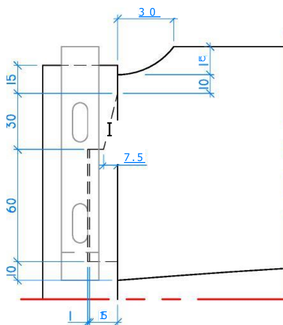
DÉTAIL 2 ÉCHELLE 1 : 2
