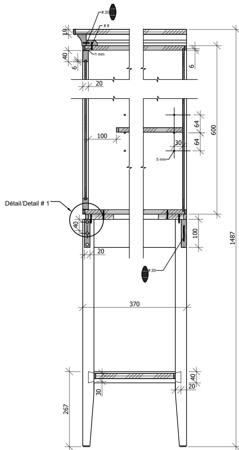
Section A-A, 1:8
