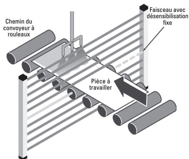
Figure 2 : Désensibilisation fixe contrôlée dans des rouleaux d'introduction.
