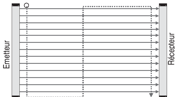
Figure 16 : Test du champ de protection avec une tige de test
