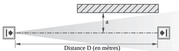
Figure 5 : Distance minimale à partir des surfaces réfléchissantes
