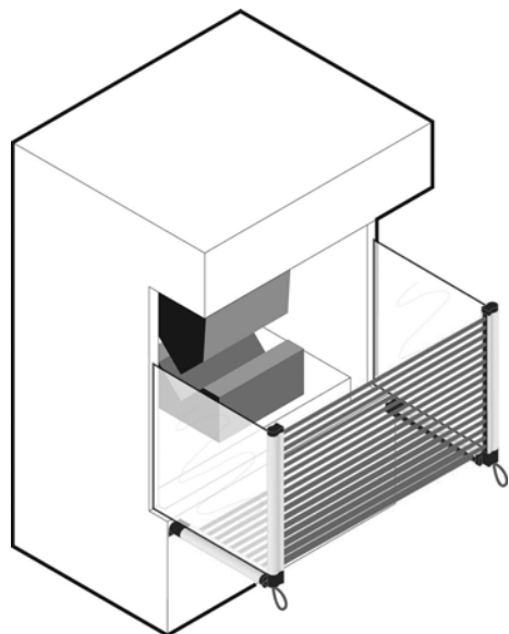
Figure 8 : Les systèmes en cascade GuardShield à deux segments « en L » offrent une protection quand il est possible de se tenir debout entre la barrière immatérielle verticale et la zone dangereuse de la machine.
