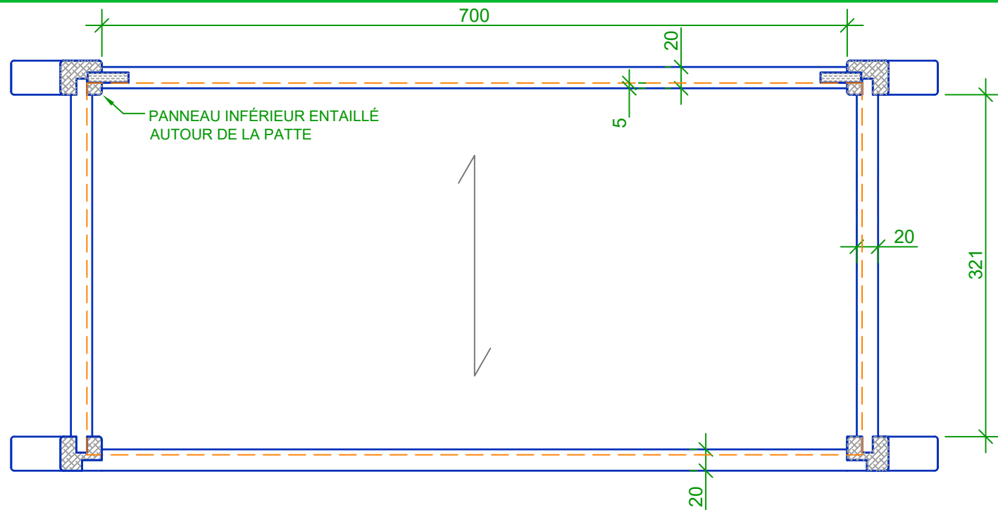
COUPE C-C
