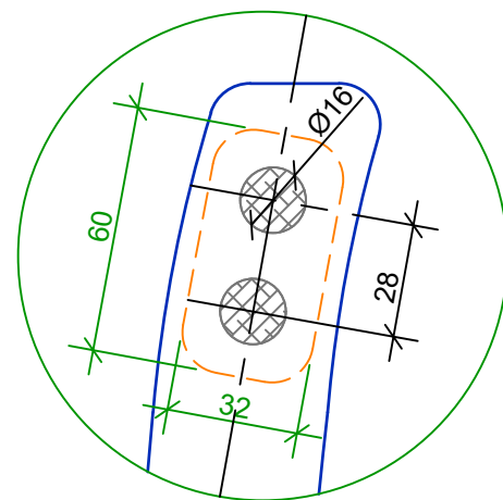
ASSEMBLAGE DE LA TRAVERSE SUPÉRIEURE - ÉCHELLE 1:2
