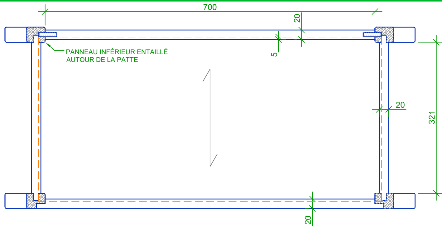
COUPE C-C
