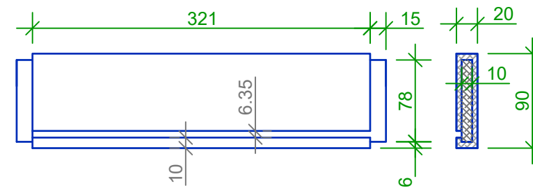
TRAVERSE DE CÔTÉ
