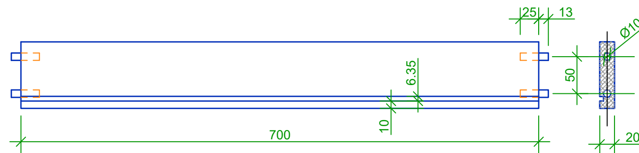
TRAVERSE ARRIÈRE
