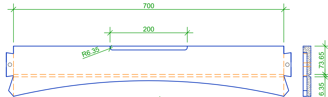
TRAVERSE AVANT À QUEUES D'ARONDE ET COUPES BIAISES
