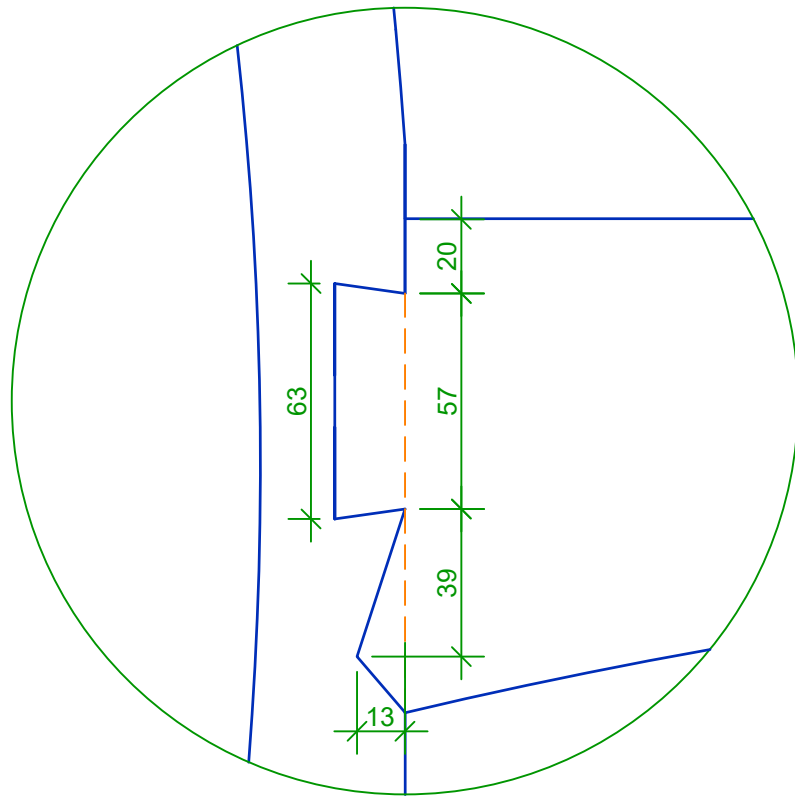
DÉTAIL QUEUE D'ARONDE AVEC COUPE BIAISE - ÉCHELLE 1:2
