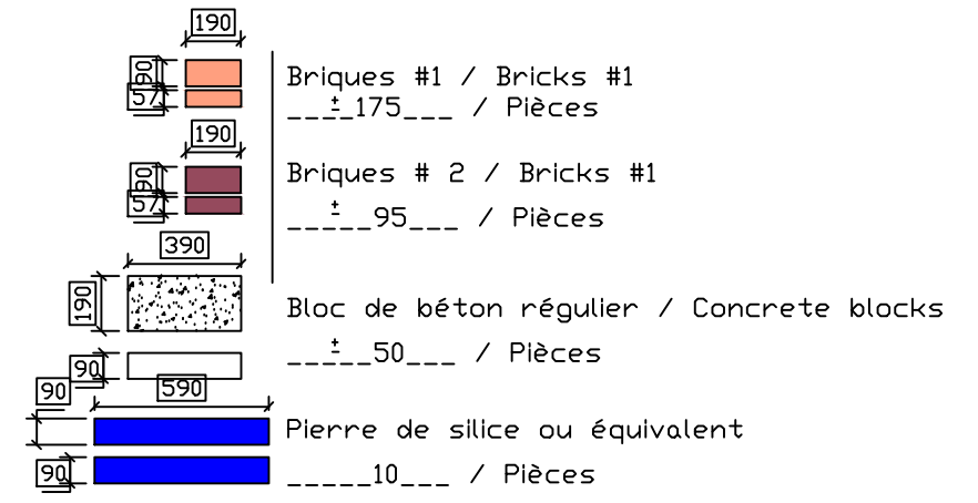
ÉLÉMENTS DE MAÇONNERIE MASONRY MATERIEL
